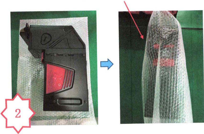
图二: 将组装好的 NV200S+NV200S CB500 V2+NV200S CB outer+PA610/PA00634 用 SPO 气泡袋包装好.
